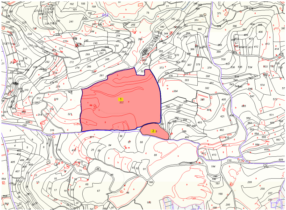
Ilustración 2: Situación Catastral de la Planta Solar Fotovoltaica
